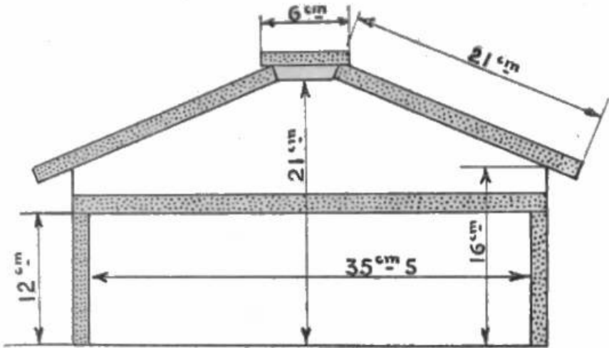
COUPE DU TOIT CHALET
