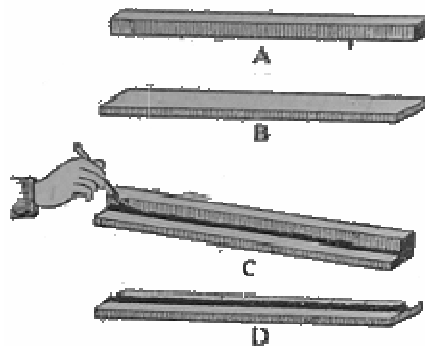
GABARIT pour amorcer les portes-rayons.
