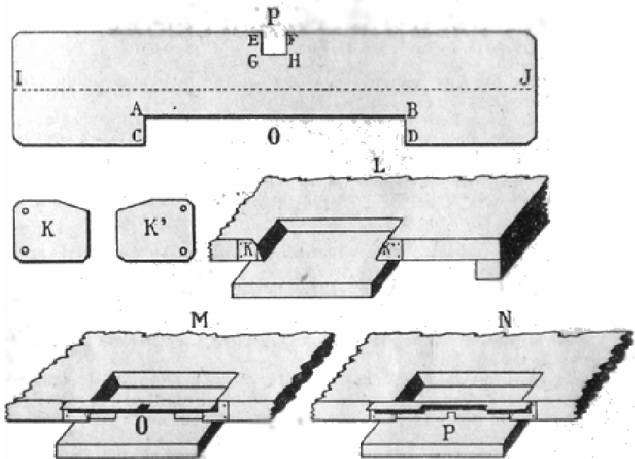
Détail de la portière.
